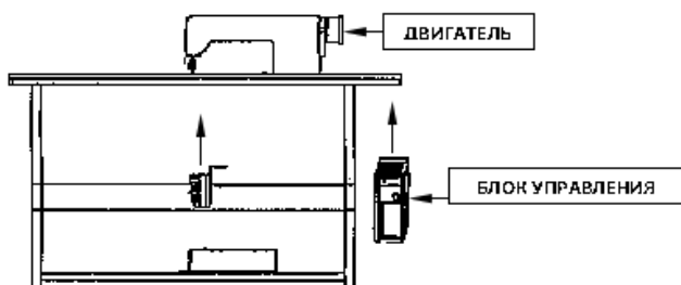
Рис. 1-3. Схема установки блока управления
