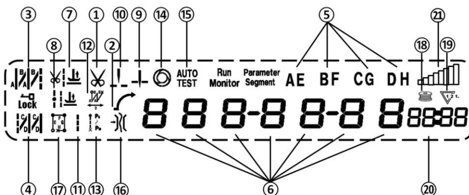
Рис. 2-4. Основные значки панели управления Н-70
