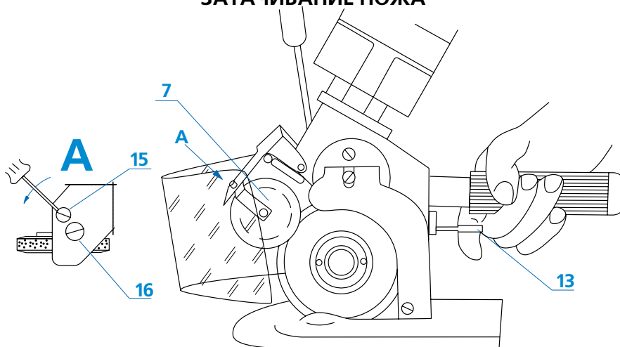
Рис. 3. Затачивание ножа.
