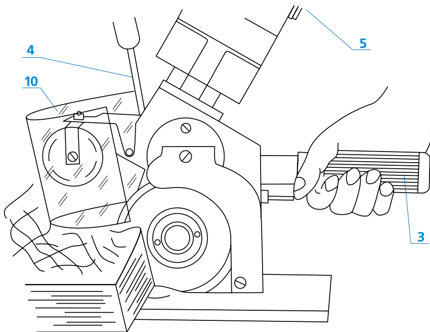
Рис. 2. Раскрой настила материала
