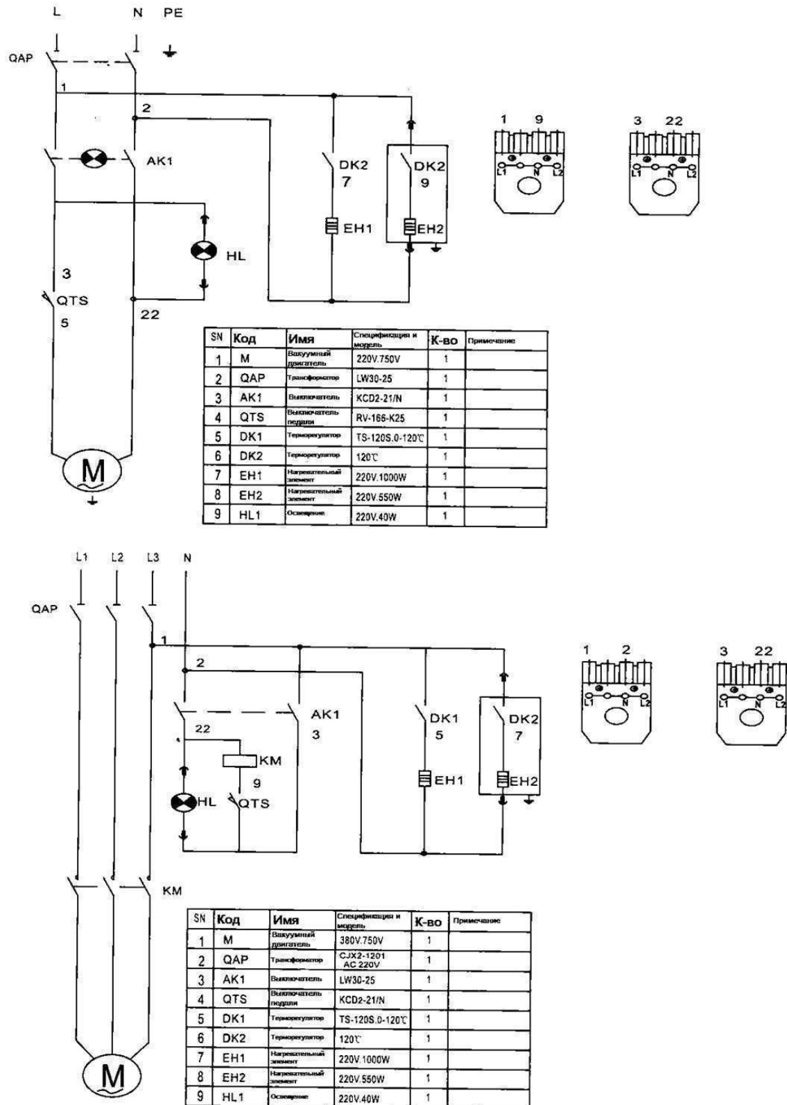
Рис. 3. Электрическая схема гладильного стола TDZ-Q1
