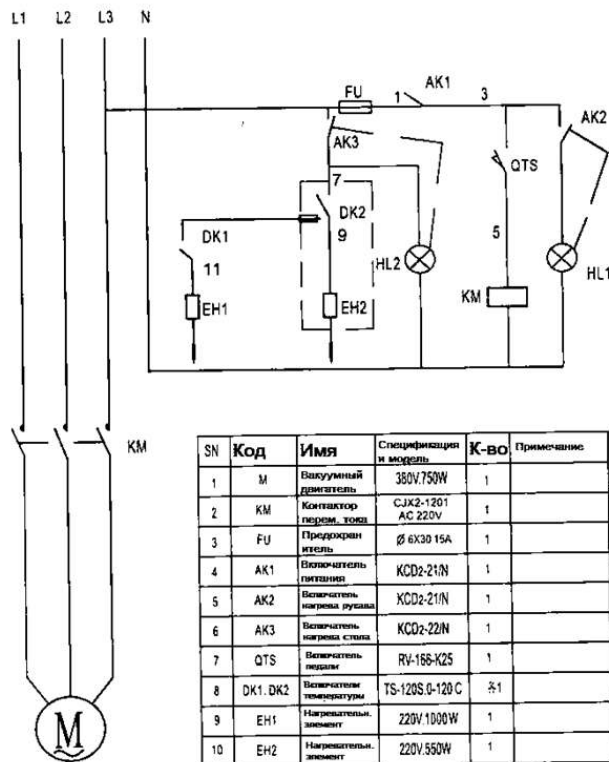
Рис. 3. Электрическая схема гладильного стола DS-TDZ-Q1
